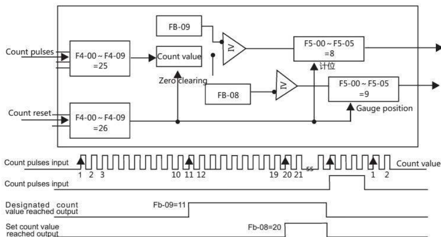
Рисунок 6-38 Достижение предельного и заданного значения счетчика
