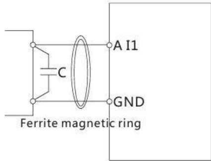
Рисунок 3-13 (ферритовое магнитное кольцо)
