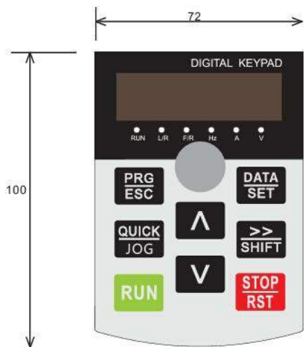
Рисунок 2-6 Внешние габариты
