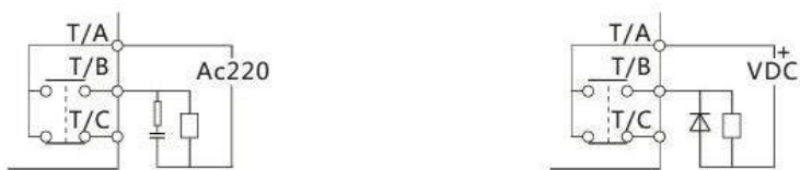
Рисунок 3-21/3-22 Внешний источник питания переменного/постоянного тока
