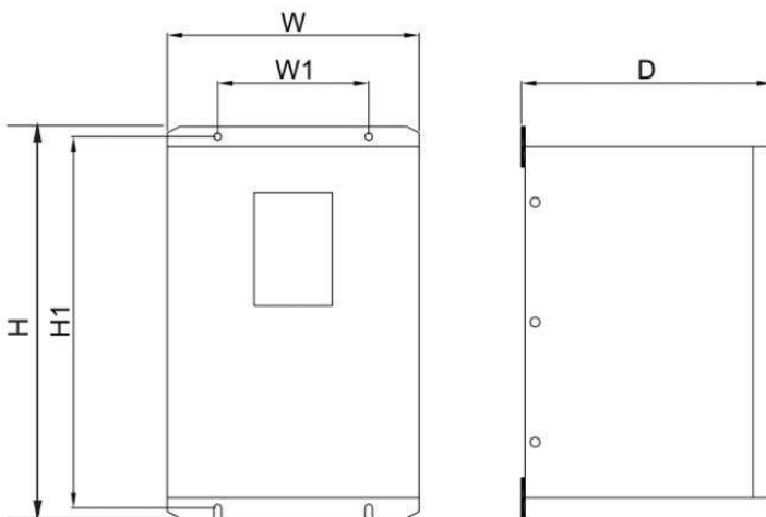
Рисунок 2-5 Внешние габариты
