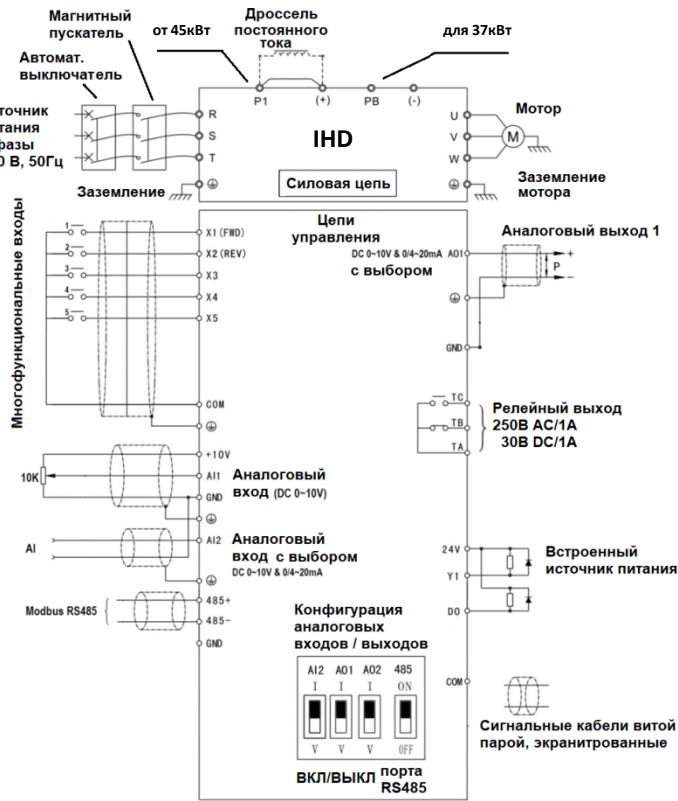
Преобразователь IHND 7,5-250 кВт
