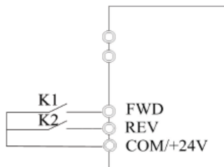
Рисунок 5-7. Двухпроводной режим работы 1 (F5-11 = 0)
