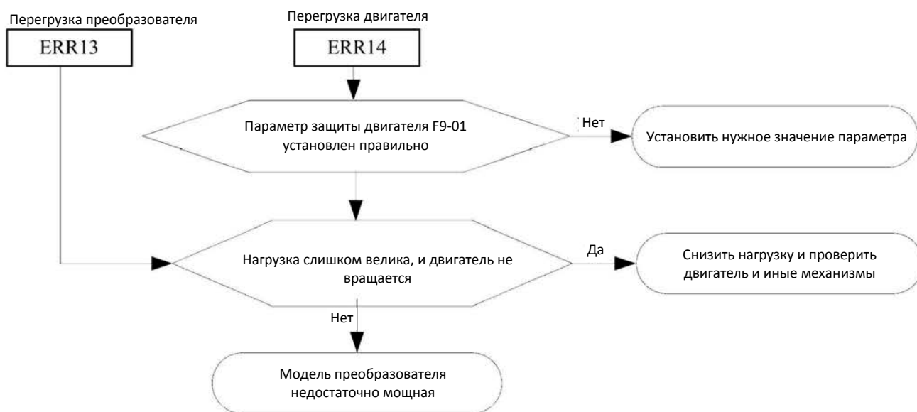
Рисунок 7-10. Перегрузка преобразователя / двигателя (Err13/Err14)
