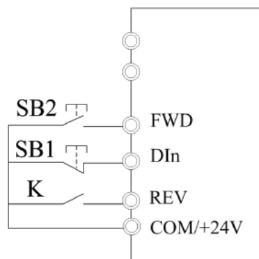
Рисунок 5-10. Трехпроводной режим работы 2 (F5-11 = 3)
