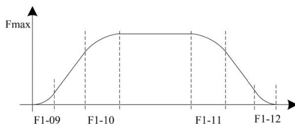
Рисунок 5-2. Диаграмма S-образного разгона и торможения
