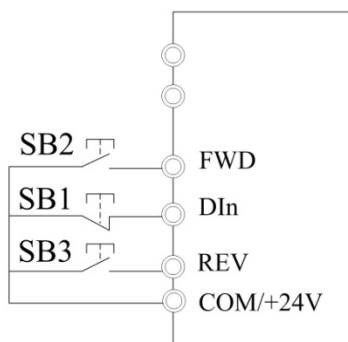
Рисунок 5-9. Трехпроводной режим работы 1 (F5-11 = 2)
