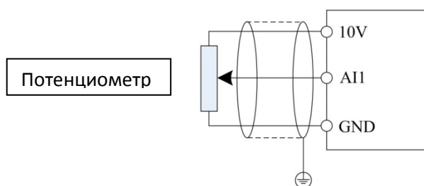
Рисунок 3-6. Схема подключения входных контактов аналогового сигнала
