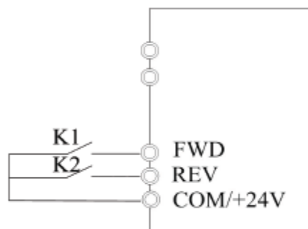
Рисунок 5-8. Двухпроводной режим работы 2 (F5-11 = 1)
