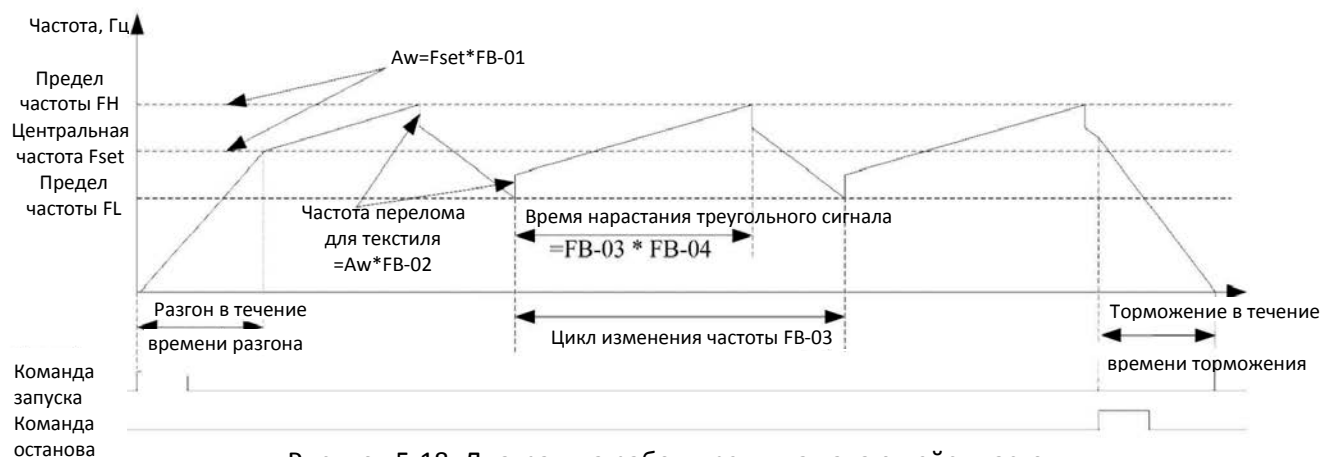
Рисунок 5-18. Диаграмма работы режима качающейся частоты
