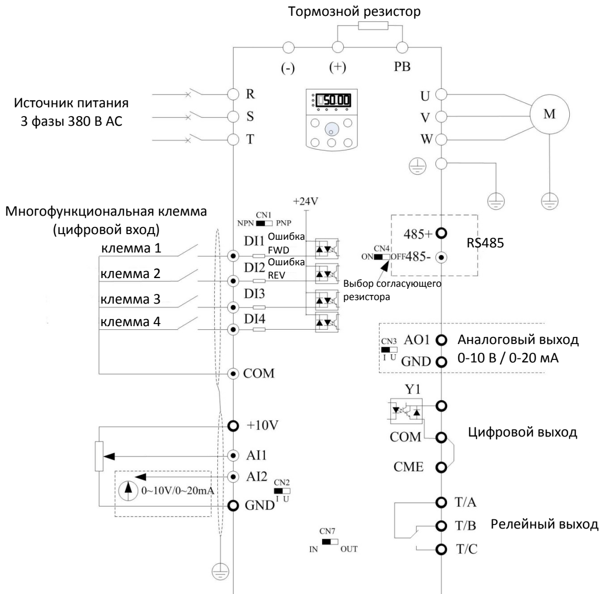
Рисунок 3-3. ADV 0.75 C420-M ~ ADV 1.50 C420-M
