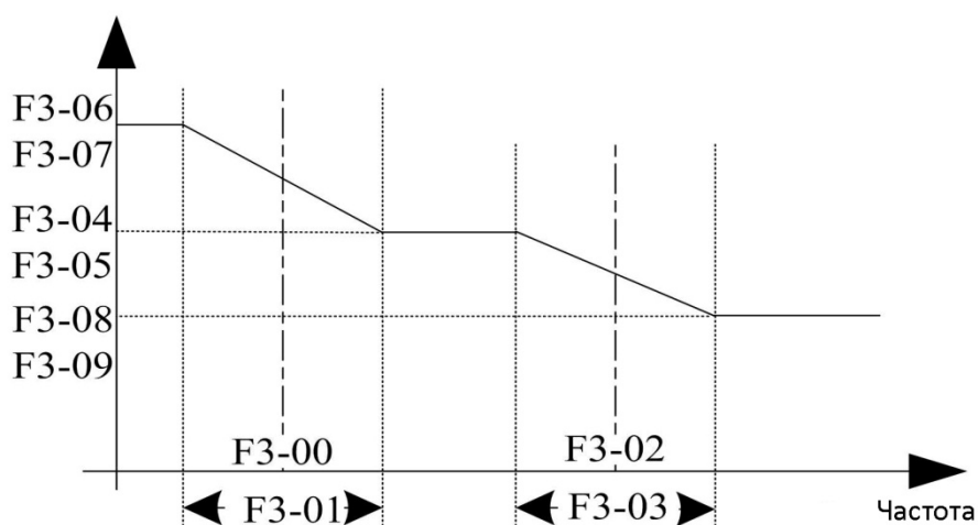
Рисунок 5-5. Схема переключения параметра PI контура управления по скорости
