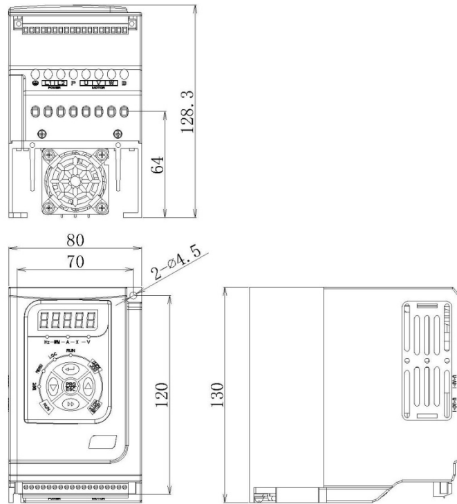
Рисунок 2-4. Габариты преобразователя и размеры монтажных отверстий
