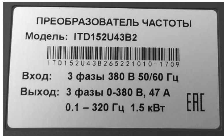
Рис.1-2 Заводская табличка продукта
