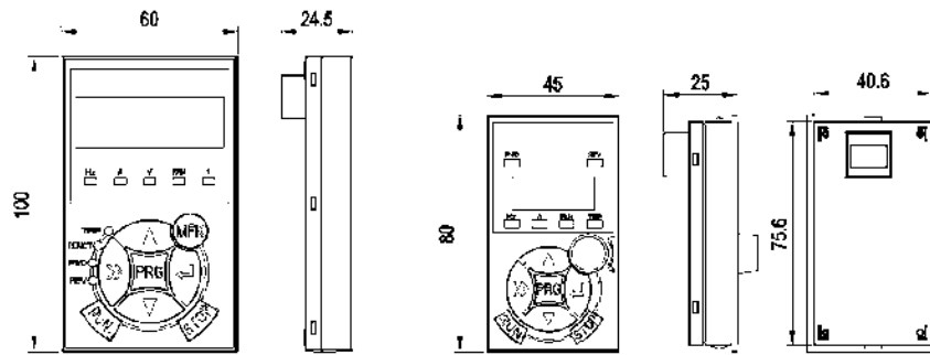
Рис.1-3 Схема пульта управления и монтажные размеры
