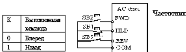
Рис.6-16 Трехпроводной режим управления 2
