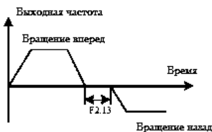
Рис. 6-6 Переключение вперед/назад
