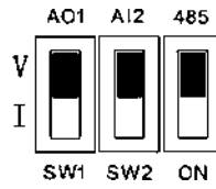
Рис. 3-17 Настройка двухпозиционного переключателя
