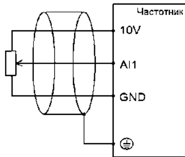
Рис. 3-14 Подключение аналоговых входов
