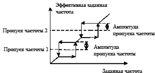
Рис. 6-5 Пропуск частот
