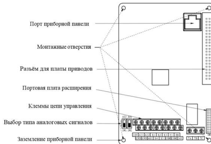
Рис. 3-16 Плата управления
