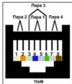
Рис. 3-15 Стандартный T568B
